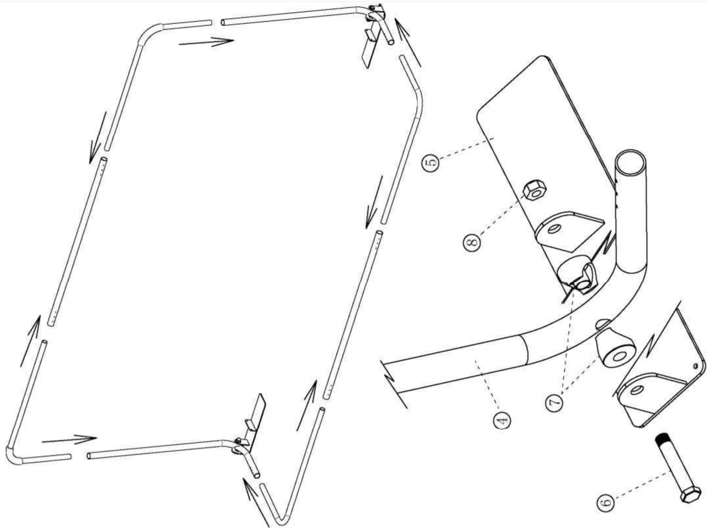
Asennuspiirros:
